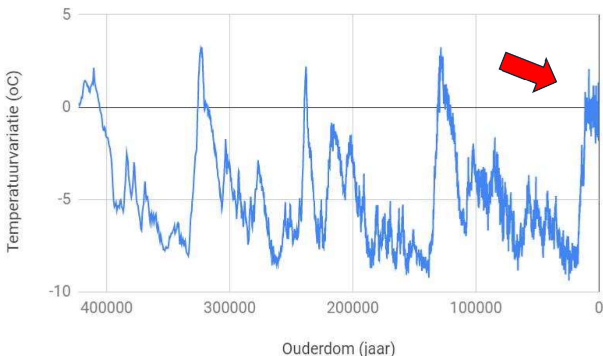
— Historische temperatuurreeks (Vostok ijsboring)
