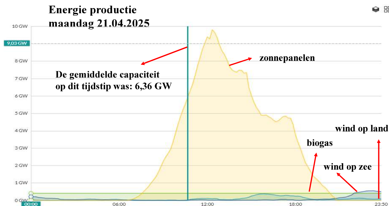
Grafiek 10 Energieopwek.nl/Entrance
