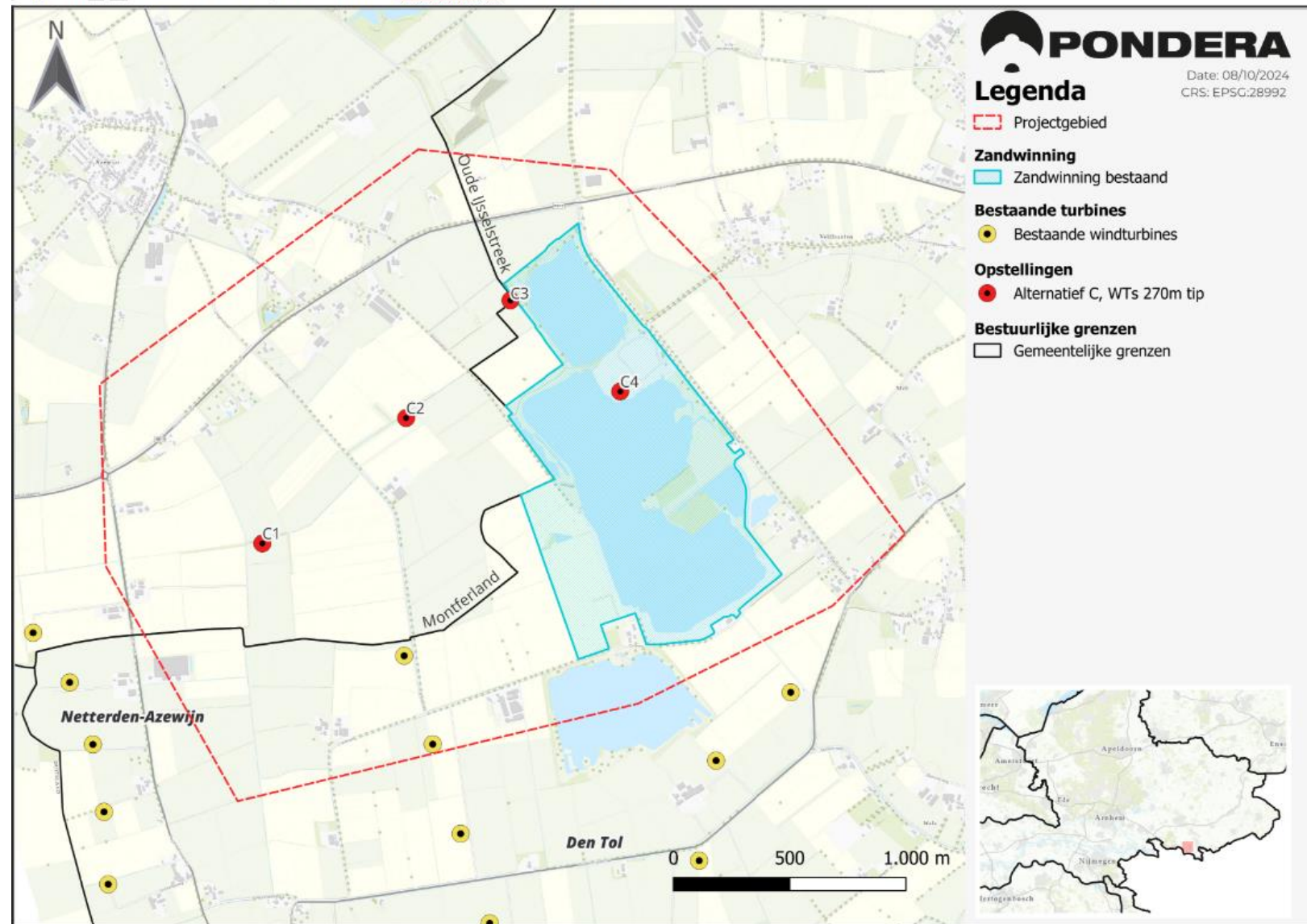
Figuur 3.6 Alternatief C, maximale tiphoogte van 270 meter
