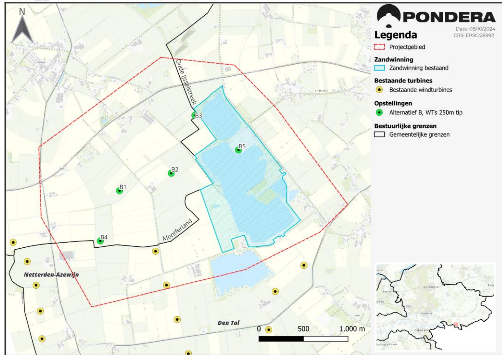
Figuur 3.5 Alternatief B, maximale tiphoogte van 250 meter
