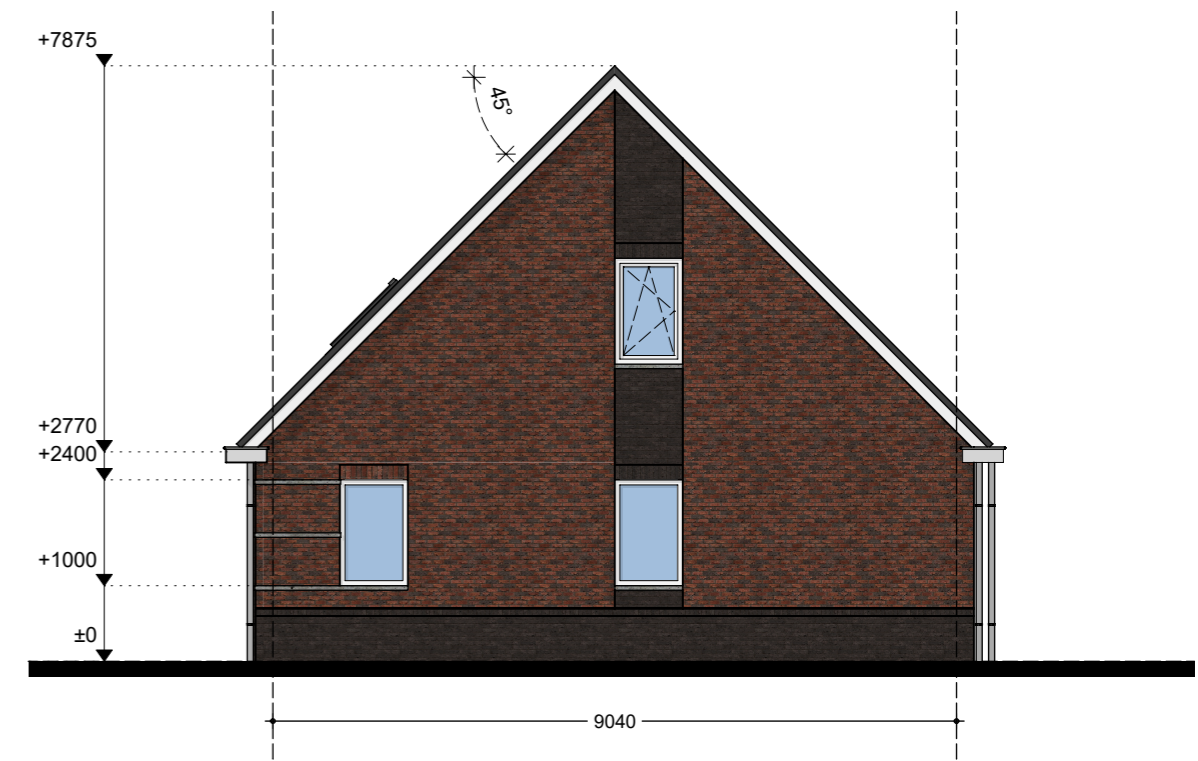
ZIJGEVEL
